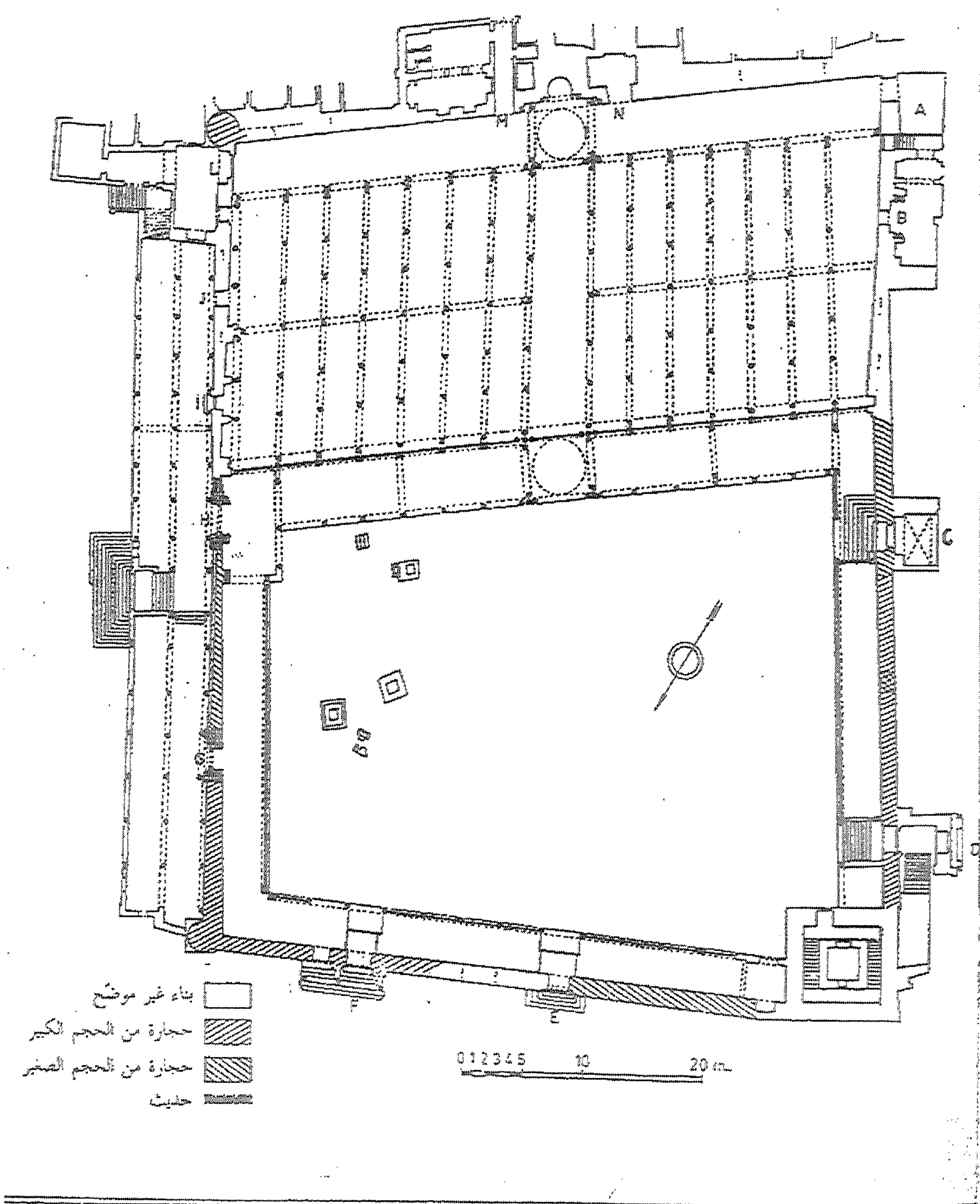
(شكل رقم ٦٦) الرسم التخطيطي الحالي لجامع الزيتونة عن جولفان .
